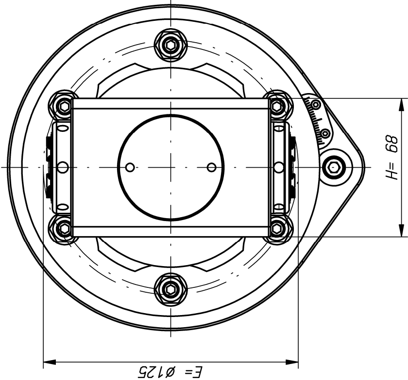
Ansicht X M1:1.5
