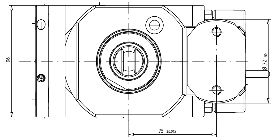
Ansicht X
