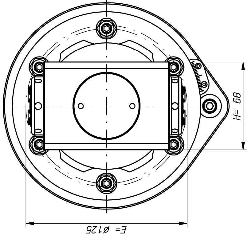
Ansicht X M1:1.5
